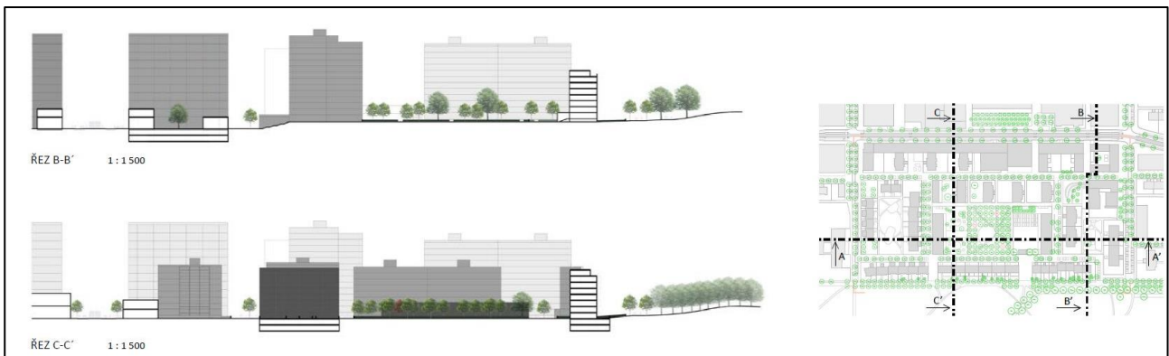
Obrázek 9: Příklad výkresu řezů územím
